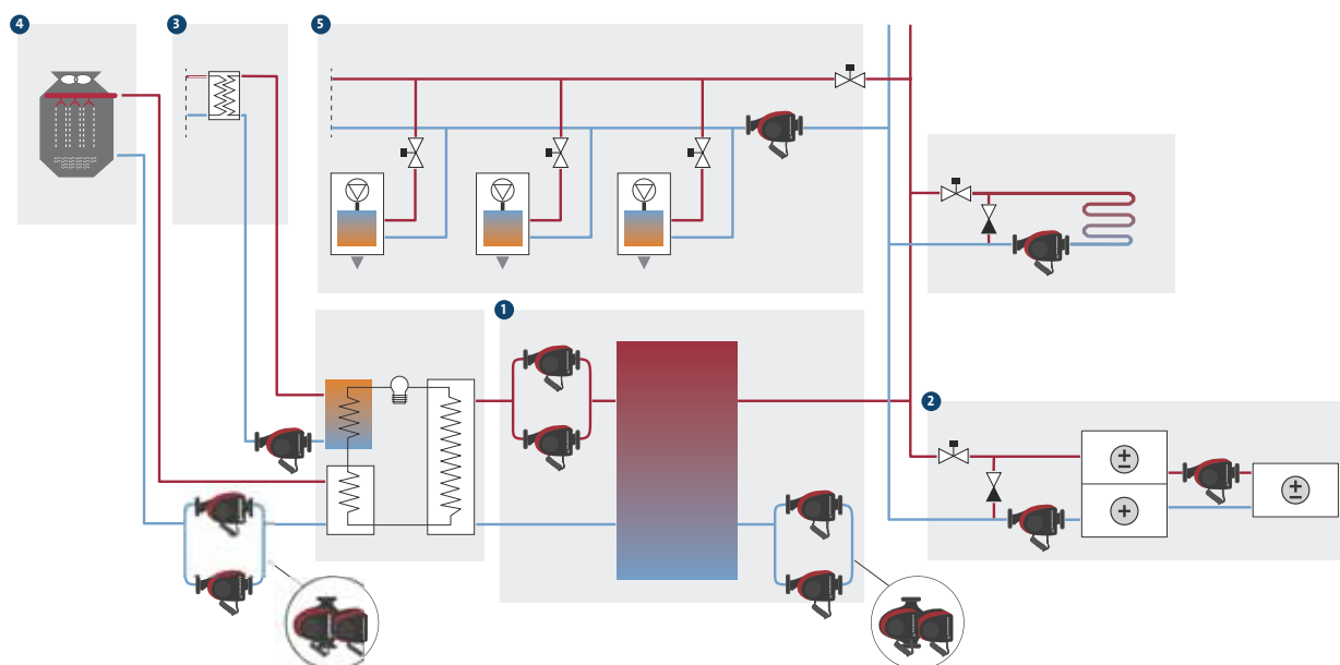
Rys. 10 Schemat funkcjonalny instalacji chłodniczej w budynku usługowo-handlowym
