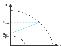
Ciśnienie proporcjonalne
