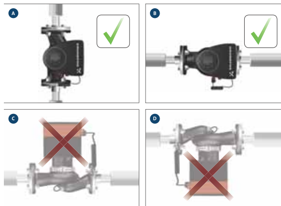
Rys. 49 Położenia montażowe
