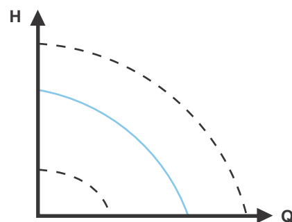
Rys. 25 Praca wg charakterystyki stałoprędkościowej
