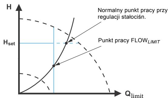
Rys. 29 Regulacja stałociśnieniowa z włączoną funkcją FLOW LIMIT
