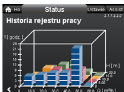
Rys. 38 Przykładowy ekran Rejestr operacyjny
