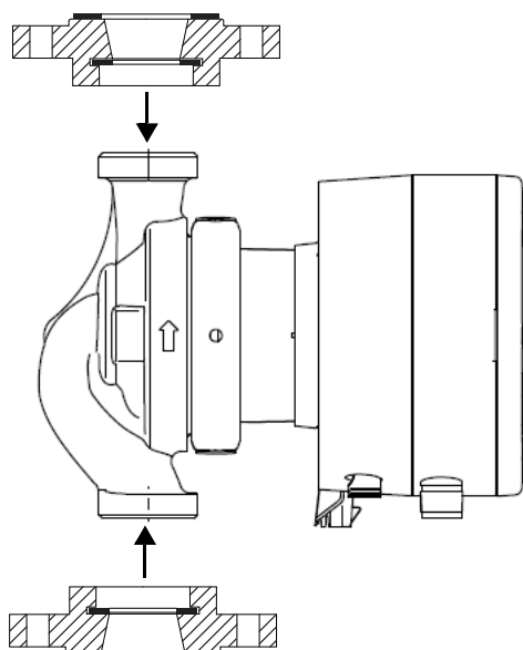
Rys. 73 Przykładowe adaptory gwint-kołnierz
