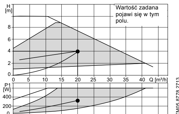
Rys. 7 Narzędzie Katalog Techniczny Grundfos Product Center (GPC)
